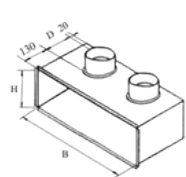
Plenum CS6 : cf. p.159
