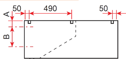
VUE LATÉRALE
