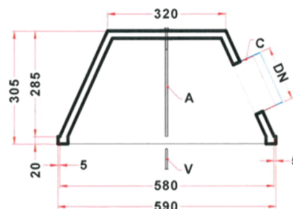
P2P : plenum polystyrène haute densité (M1)
