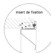
Contre cadre CTP : cf. p.150
