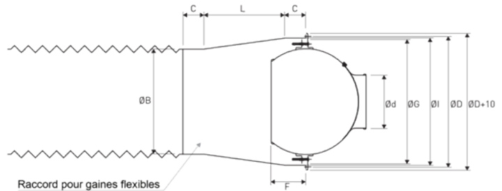
Montage sur gaine flexible avec le raccord KDVTR
