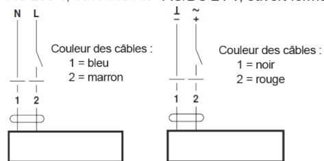
Câblage LF230
