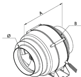
Ø 125, 160, 160L, 200, 200L
