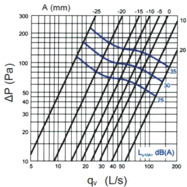
LK Ø200
