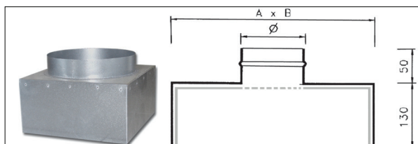
Plenum de soufflage en tôle d'acier galvanisé isolé
