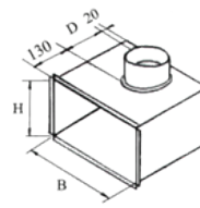
Plenum CS4 : cf. p.157
