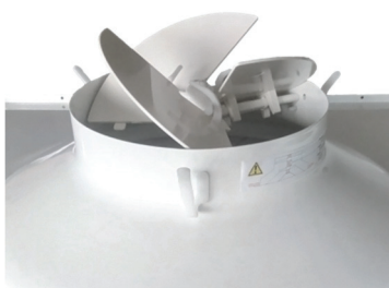
Registre réglable
