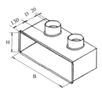
Plenum CS6 : cf. p.159
