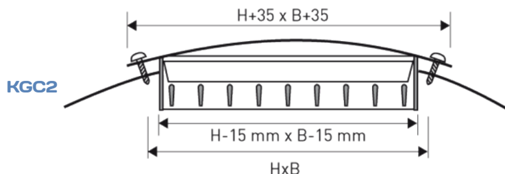
Dimensions et débits d'air
