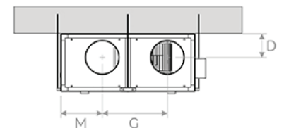
Vue arrière
