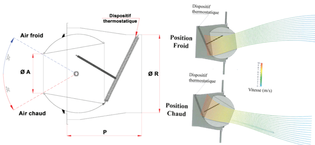
Dimensions modèle et débits d'air
