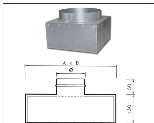
Plenum isolé DP1IS de soufflage
