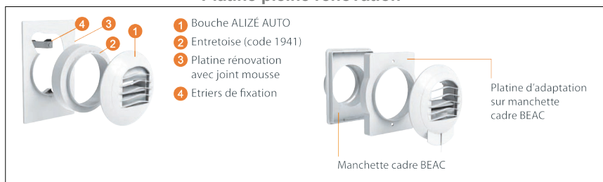
Platine pleine rénovation
