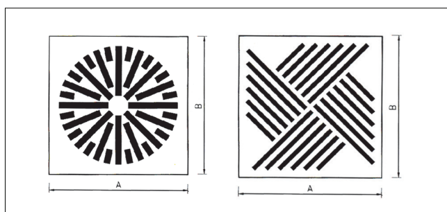
Dimensions et débit d'air : KDAFP et KDBFP
