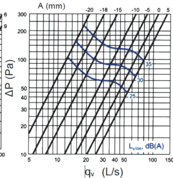
LK Ø160
